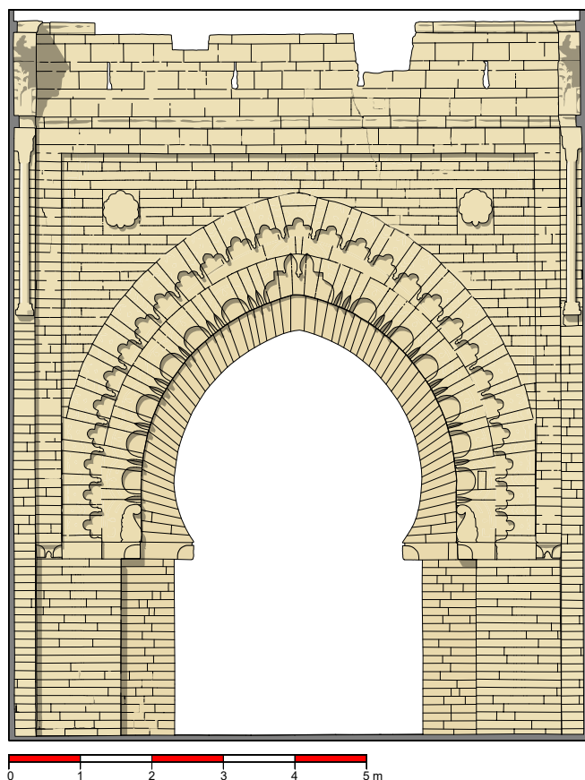
Figure 17. Stéréotomie et découpage de l'appareil en pierre de taille de la façade extérieure de la porte d'apparat de Šālla (© Les auteurs).
