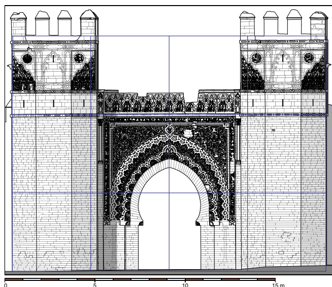
Figure 13. Rectangle pythagoricien (4/3) régissant l'élévation de la porte d'apparat de Šālla et de ses tours de flanquement (© Les auteurs).
