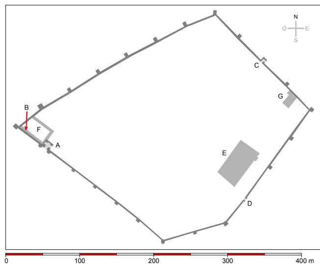
Figure 1. Plan général de l'enceinte de Šālla et des principaux ensembles monumentaux médiévaux qu'elle enferme. A. Porte d'apparat (accès principal) ; B. Emplacement de l'épure architecturale mérinide étudiée dans cet article ; C. Bāb 'Ayn Aḡanna ; D. Bāb al-Basātīn ; E. Halwa , complexe religieux et funéraire ; F. Funduq ; G. Hammām (© Les auteurs).
