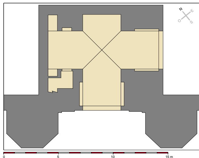
Figure 9. Porte d'apparat de Šalla. Plan simplifié (© Les auteurs).
