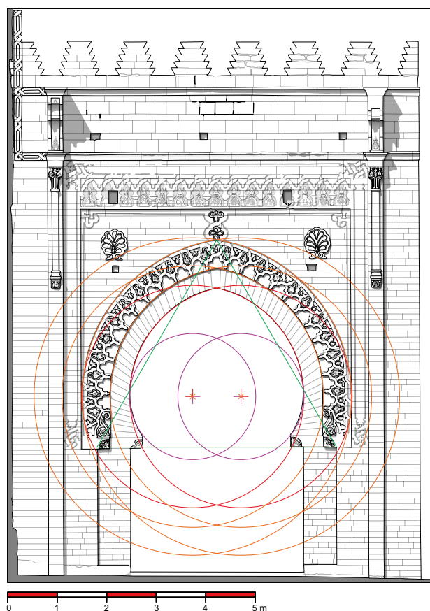
Figure 28. Schéma directeur de la façade intérieure de la porte d'aparat de Šālla (© Les auteurs).
