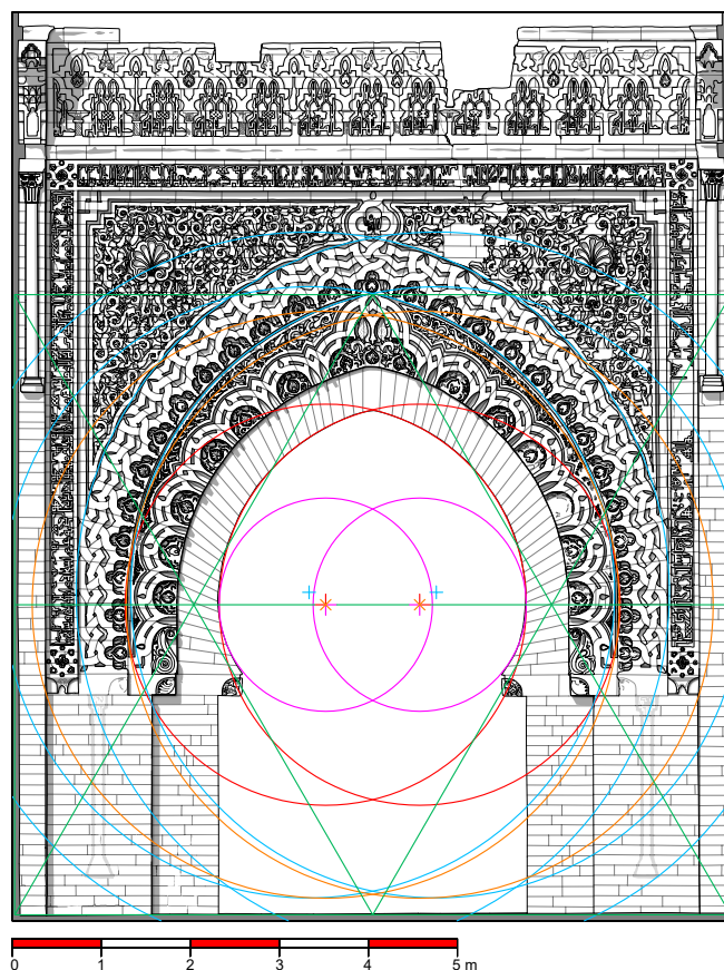
Figure 16. Schéma directeur et tracé géométrique des divers arcs de la façade extérieure de la porte d'apparat de Šālla (© Les auteurs).
