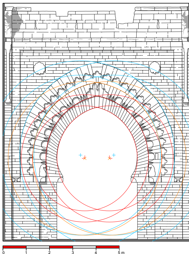
Figure 18. Schéma directeur et tracé géométrique des voûtures des arcs de la façade extérieure de la porte d'apparat de Šālla (© Les auteurs).
