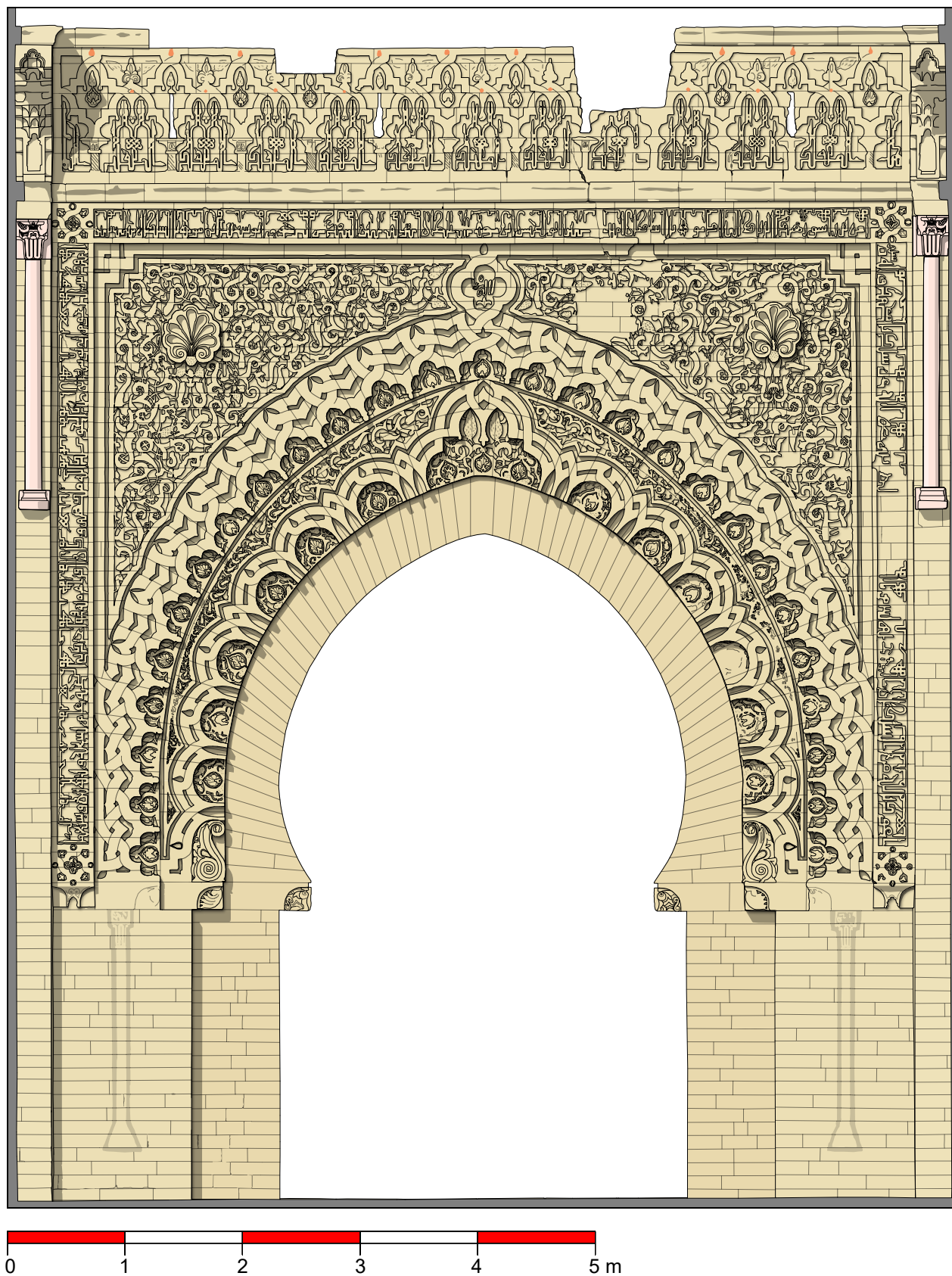
Figure 7. Relevé photogrammétrique de la façade extérieure de la porte d'apparat de Šālla (© Les auteurs).
