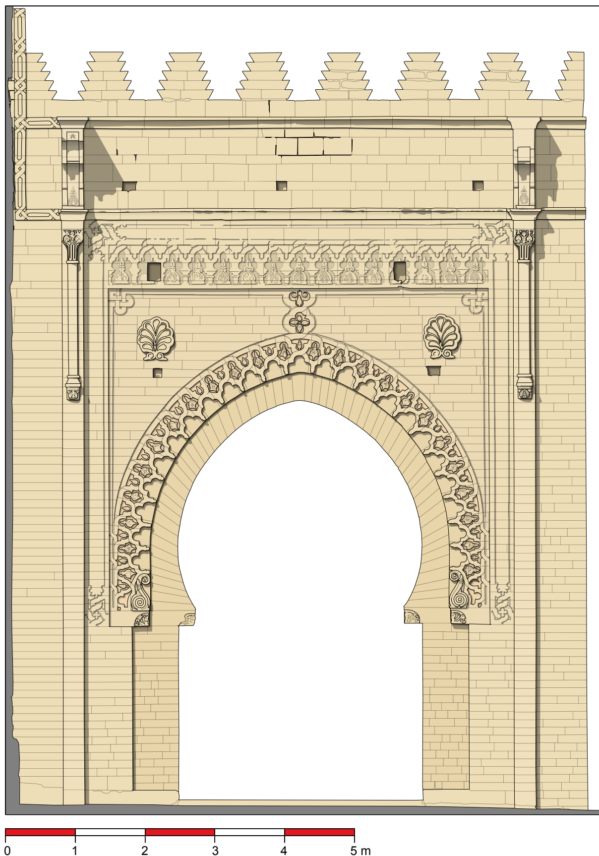
Figure 26. Relevé photogrammétrique de la façade intérieure de la porte d'apparat de Šālla (© Les auteurs).
