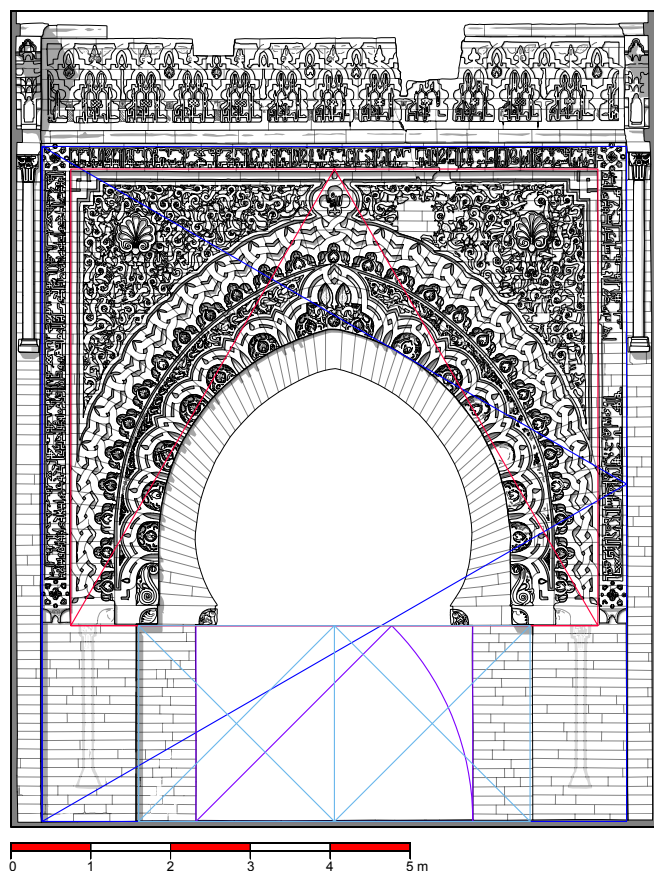
Figure 15. Schéma directeur de la façade extérieure de la porte d'apparat de Šālla (© Les auteurs).
