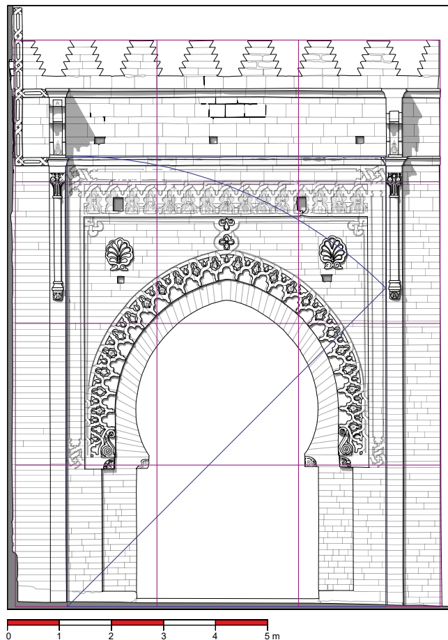
Figure 27. Schéma régulateur de la façade intérieure de la porte d'apparat de Šalla (© Les auteurs).
