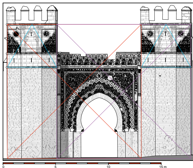
Figure 14. Schéma directeur de l'élévation de la porte d'apparat de Šālla et de ses tours de flanquement (© Les auteurs).
