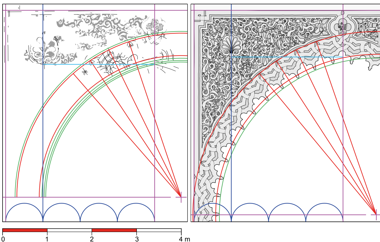
Figure 33. Analyse comparative des schémas régulateurs de l'épure et de la façade extérieure de la porte d'apparat de Šālla (© Les auteurs).
