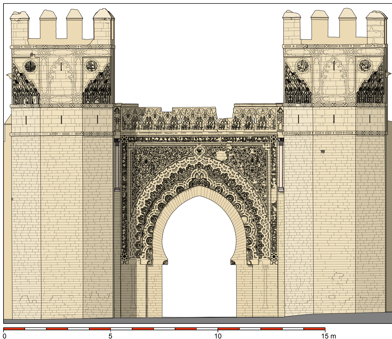
Figure 11. Relevé photogrammétrique de la façade extérieure de la porte d'apparat de Šālla et des tours de flanquement (© Les auteurs).
